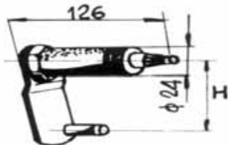
Art. 45.0053 Rif. Orig. 0050566. PERNO TERGI SX 201 MENARINI
