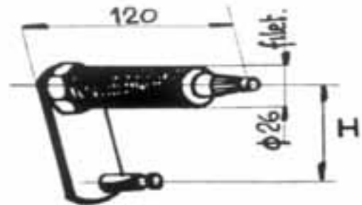
Art. 45.0121 Rif. Orig. 0646117 PERNO TERGI DX H=83/84 F1 101MN
