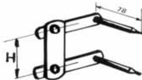
Art. 45.0078 Rif. Orig. 9980431 PERNO TERGI 370.26
