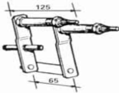
Art. 45.0037 Rif. Orig. 0053400. PERNO TANDEM DX 201 MN
