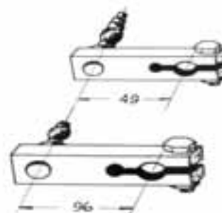
Art. 45.0095 SERIE MANOVELLE L=49 L=96
