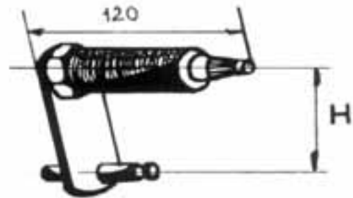
Art. 45.0122 Rif. Orig. 8123147 PERNO TERGI SX H=68 F1 101MN
