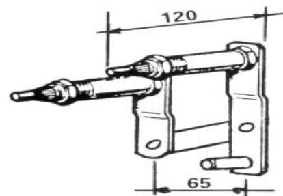
Art. 45.0073 Rif. Orig. 0057239. PERNO TANDEM DX-SX 201 MN
