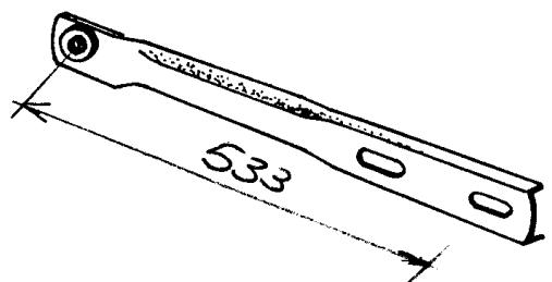
Art. 45.0195 BIELLA CENTRALE REGOL.AZIONE MACCHI 418 FILOSOD
