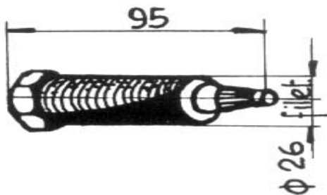
Art. 45.0112 Rif. Orig. 8193889 PERNO CENTRALE FOLLE 480
