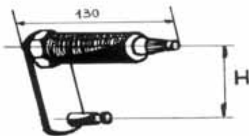
Art. 45.0085 Rif. Orig. 8194076 PERNO TERGI H=70mm. 370R Art. 45.0086 Rif. Orig. 42485027 PERNO TERGI H=88mm. 370R
