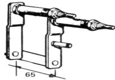
Art. 45.0038 Rif. Orig. 0053401. PERNO TANDEM SX 201 MN
