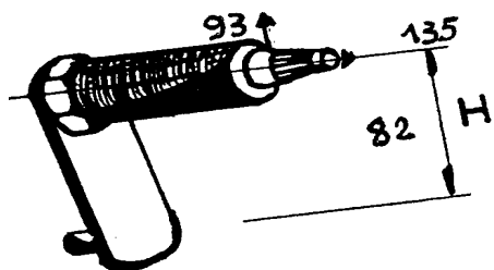
Art. 45.0185 PERNO TERGI DX BUSOTTO
